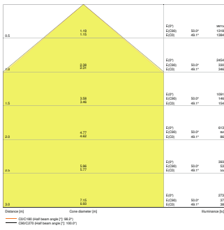
FL PFM 50W4000K SYM 100 S BK
