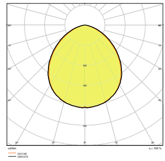
FL PFM 50W4000K SYM 100 S BK
