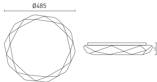
LD-STARS48W-NW-00
